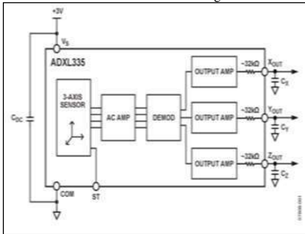
Fig. 5: Accelerometer
