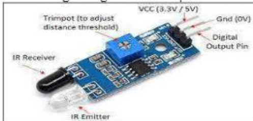
Fig 5. IR sensor
