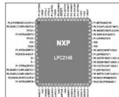
Fig 3. ARM (LPC2148)
