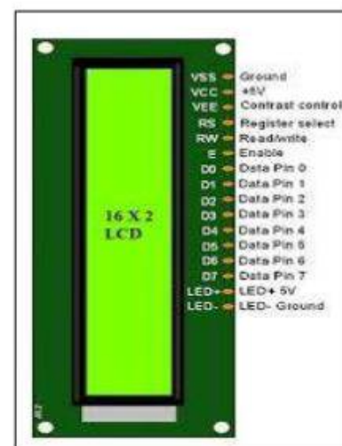
Fig 3.3. LCD 16X2
