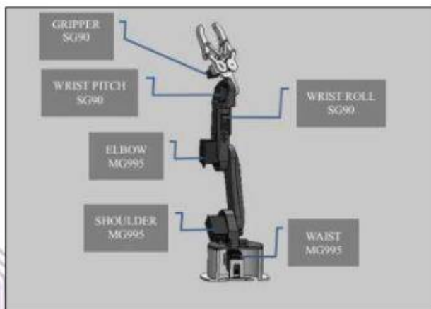
Fig. 3.3 Robotic arm
