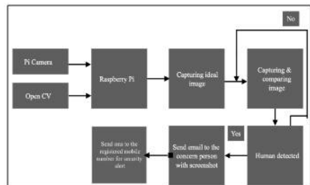
Fig 2.5. open cv
