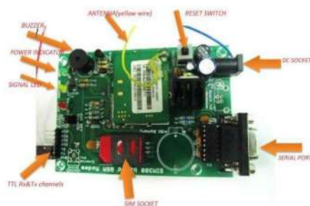
Fig. 3 GSM MODEM
